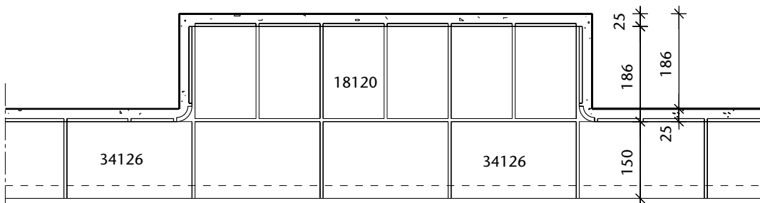
Schnitt B-B/Coupe B-B/Section B-B/Sezione B-B
