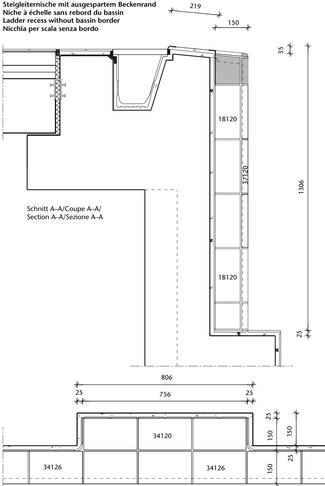
Schnitt B-B/Coupe B-B/Section B-B/Sezione B-B
