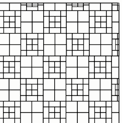
Malli 11 3 kokoa suhteissa 50:25:25, esim. 20x20cm, 10x20cm & 5x5cm Malli 12 2 kokoa suhteessa 50:50, esim. 10x10cm & 5x5cm tai 90x90cm & 45x45cm Malli 13 3 kokoa suhteessa 57,1:28,6:14,3, esim. 20x20cm, 10x20cm & 10x10cm Malli 14 1 koko Malli 15 3 kokoa suhteissa 53:23,5:23,5, esim. 30x30cm, 20x20cm & 10x20cm
