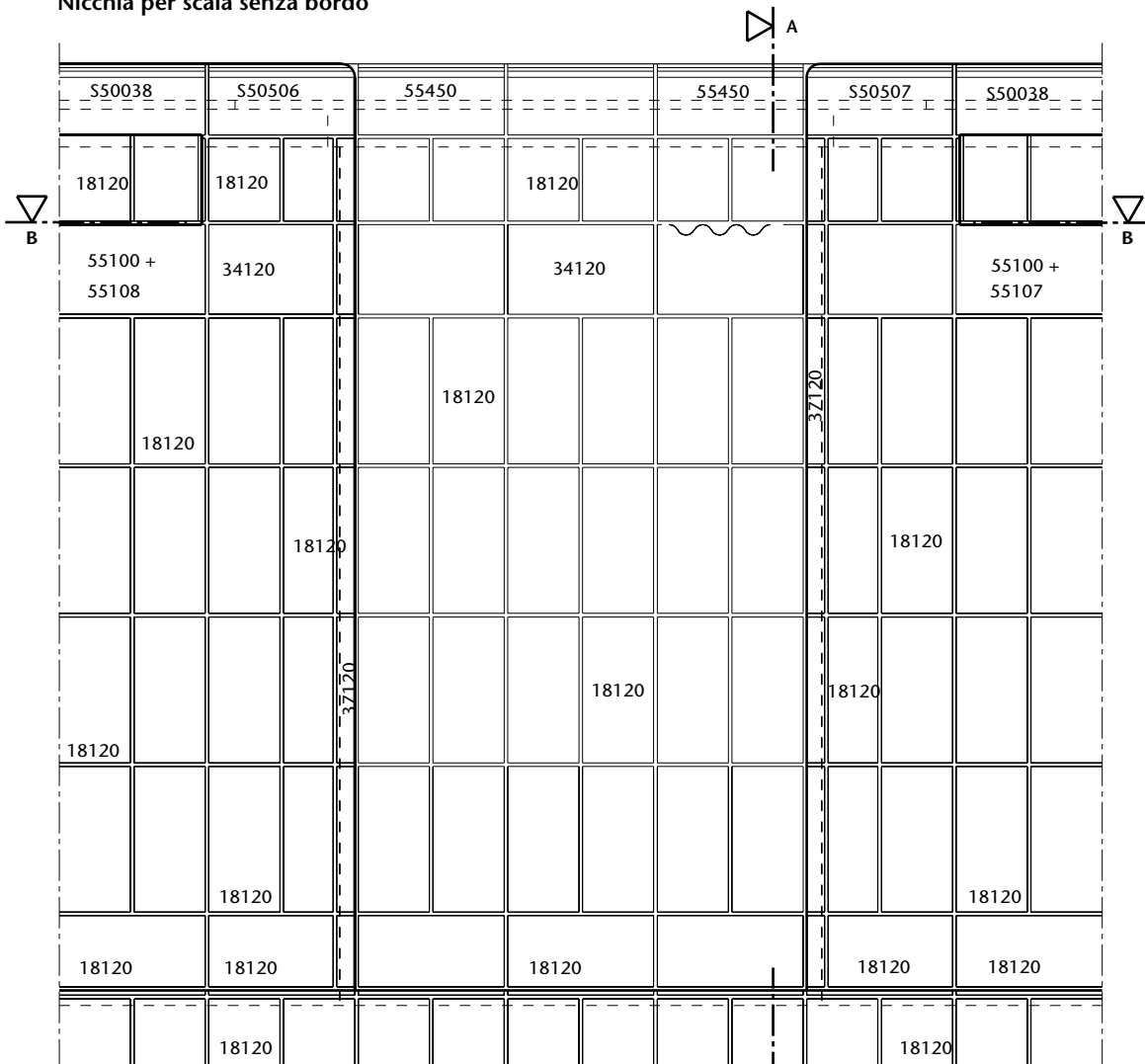
Ansicht/Vue/View/Vista
